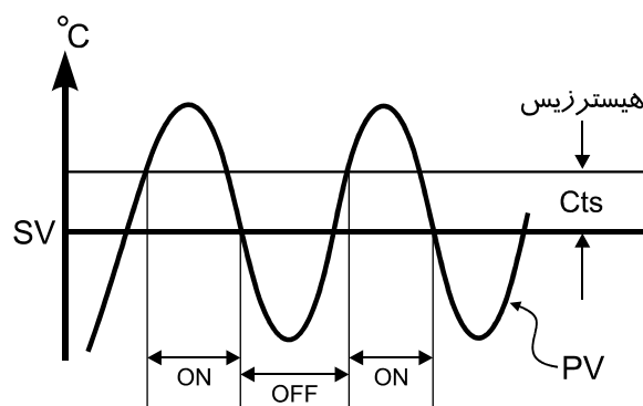
کنترل روشن / خاموش (ON/OFF) "سرد کننده"
